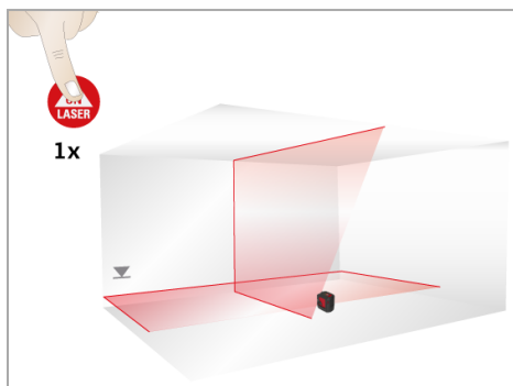
Linee laser orizzontali e verticali attive
